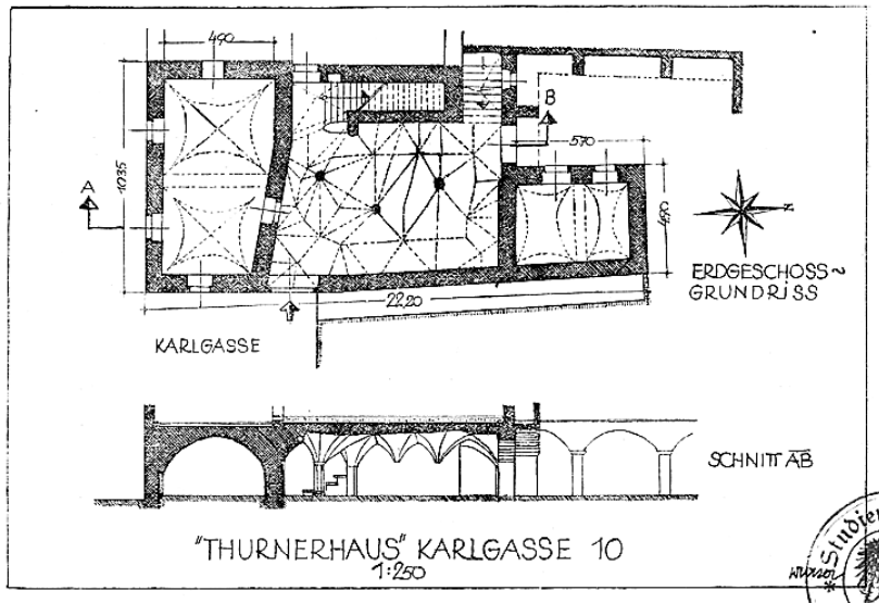
Abb. 2: Das Thurnerhaus in Villach Planzeichnung nach Rudolf Wurzer (1948)
