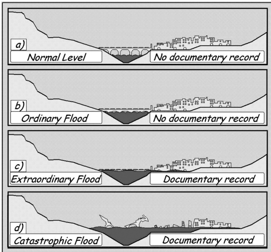
Abb. 3: Schematische Darstellung von Kriterien zur Festlegung unterschiedlicher Überschwemmungen. Hierbei wird besonderer Bezug auf die Verfügbarkeit von historischen Daten gelegt Llasat u. Barriendos 2001
