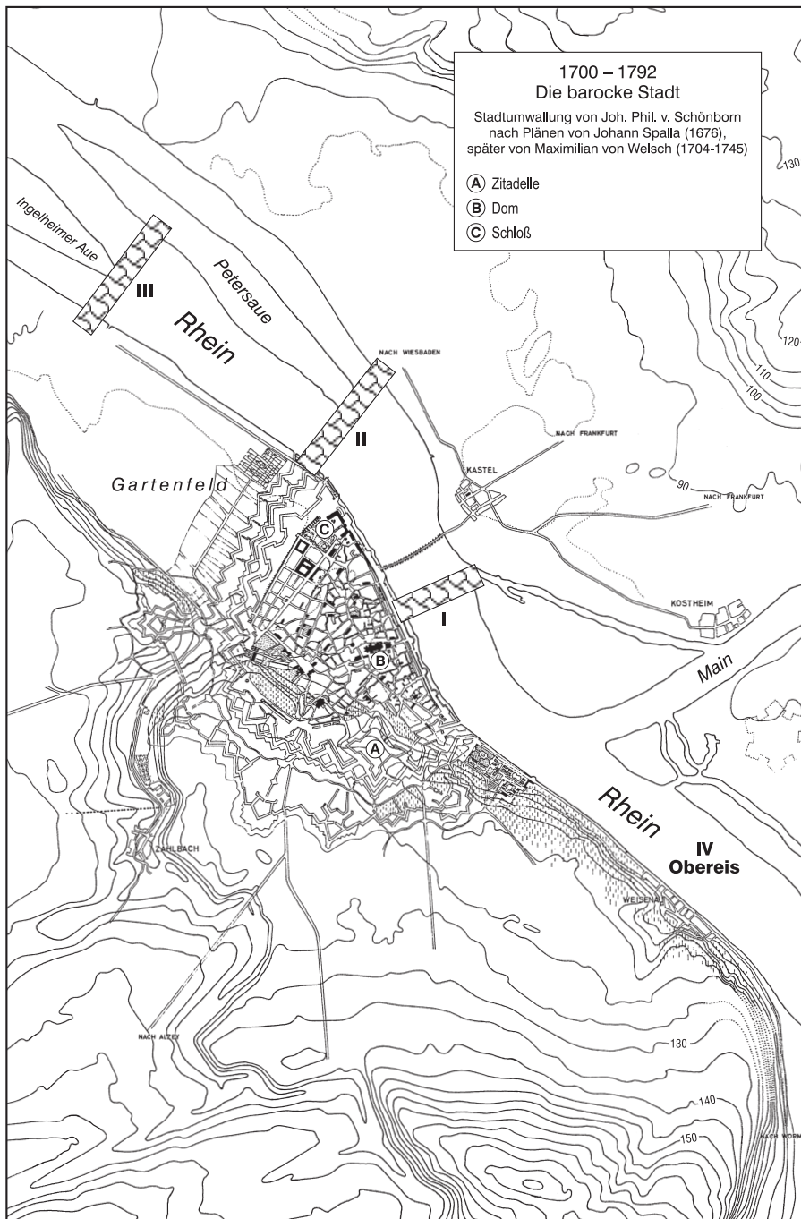
Abb. 3: I, II, III, IV: Phasen und Eisbarrieren der Hochwasserkatastrophe von 1784 in Mainz
