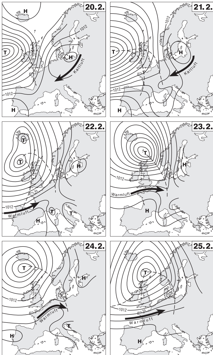
Abb. 2: Luftdruckverteilung (Wetterlagen) über Europa vom 20–25. Februar 1784 Quelle: Kingston 1988; Hauptwindrichtungen der Kalt- und Warmluft ergänzt
