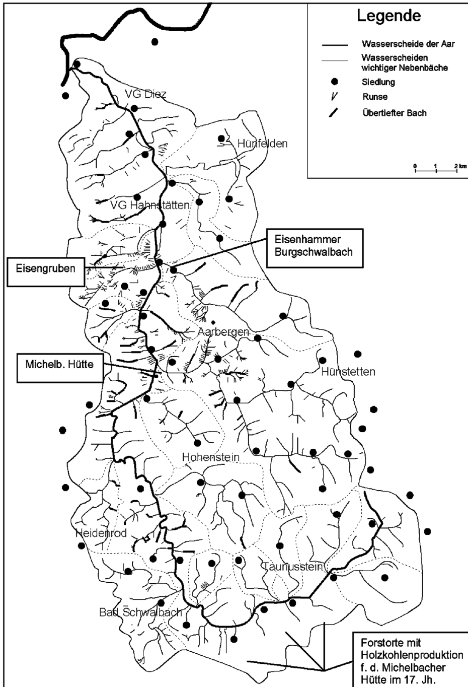
Abb. 3: Verbreitung der Runsen im Wassereinzugsgebiet der Aar
