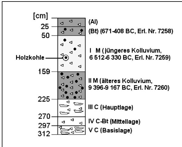
Abb. 12: Aufschluss SWA15-C2/3 am Unterlauf der Runse bei Bad Schwalbach
