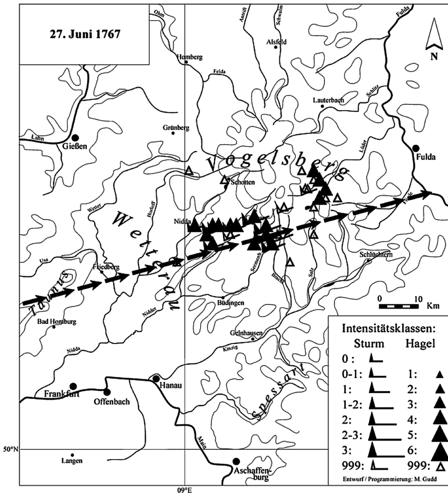
Abb. 1.: Das Schwergewitter vom 27. Juni 1767 – Verlauf und Schäden Quelle: Gudd 2004, S. 460, verändert
