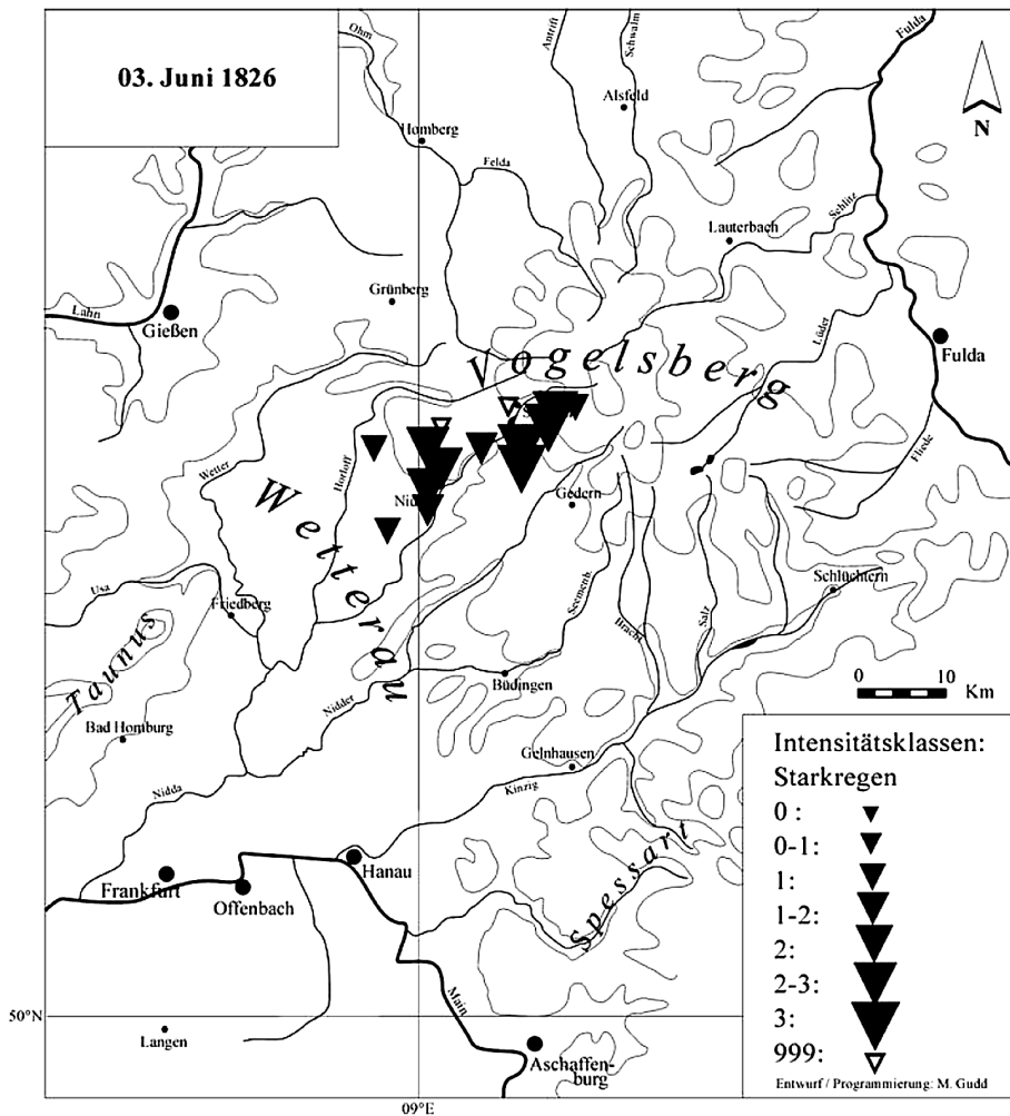
Abb. 3.: Der Wolkenbruch vom 03. Juni 1826 – Verlauf und Schäden
