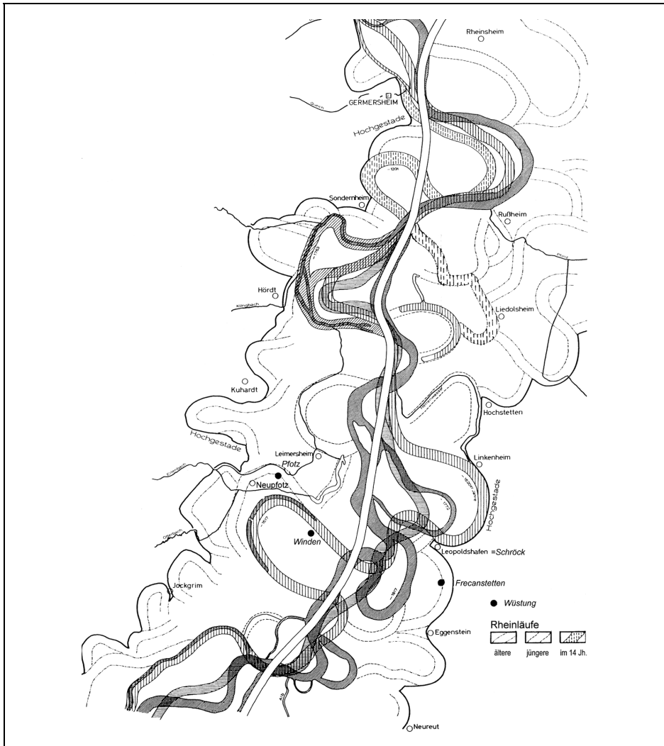
Abb. 2: Historische Veränderungen des Rheinlaufs zwischen Karlsruhe und Speyer überarbeitet nach H. Musall 1969, Maßstab 1:140.000
