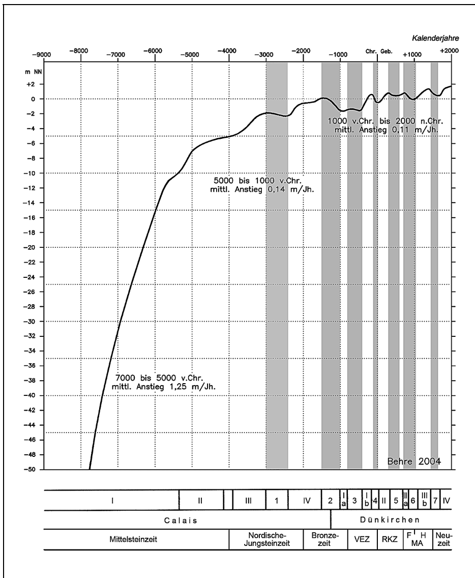
Abb. 1: Meeresspiegelkurve für die südliche Nordsee. Zeitangabe in kalibrierten Kalenderjahren. In der Fußleiste sind die Transgressionen mit römischen, die Regressionen mit arabischen Ziffern angegeben.
