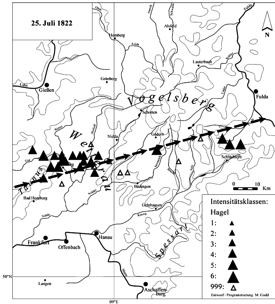
Abb. 2.: Das Schergewitter vom 25. Juli 1822 – Verlauf und Schäden Quelle: Gudd 2004, S. 466, verändert
