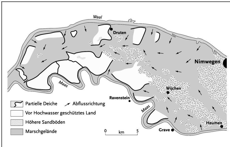
Abb. 5: Partielle Deiche im Flussbereich zwischen Waal und Maas westlich von Nimwegen (nach Van de Ven 2003, S. 92)
